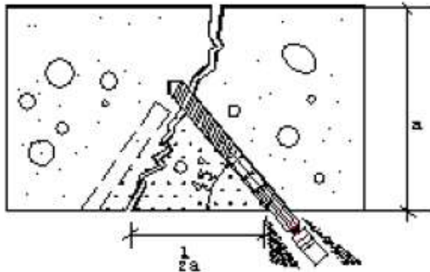
ลักษณะองศาที่เสียบรอยร้าว The degree of plug in packer to crack
