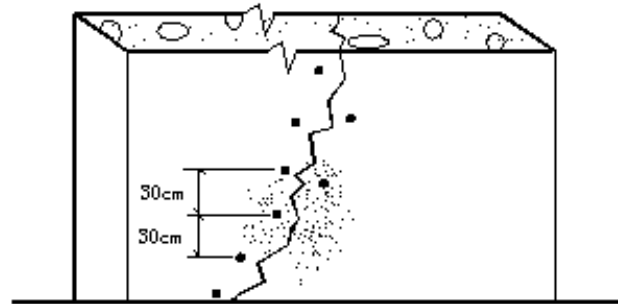
ระยะห่าง โดยทั่วไประหว่างจุดเสียบแพคเกอร์อยู่ที่ ทุก ๆ ระยะห่าง 30 ซม. แต่ต้องขึ้นอยู่กับหน้างาน The location of packer will apart 30 cm along size the crack.
