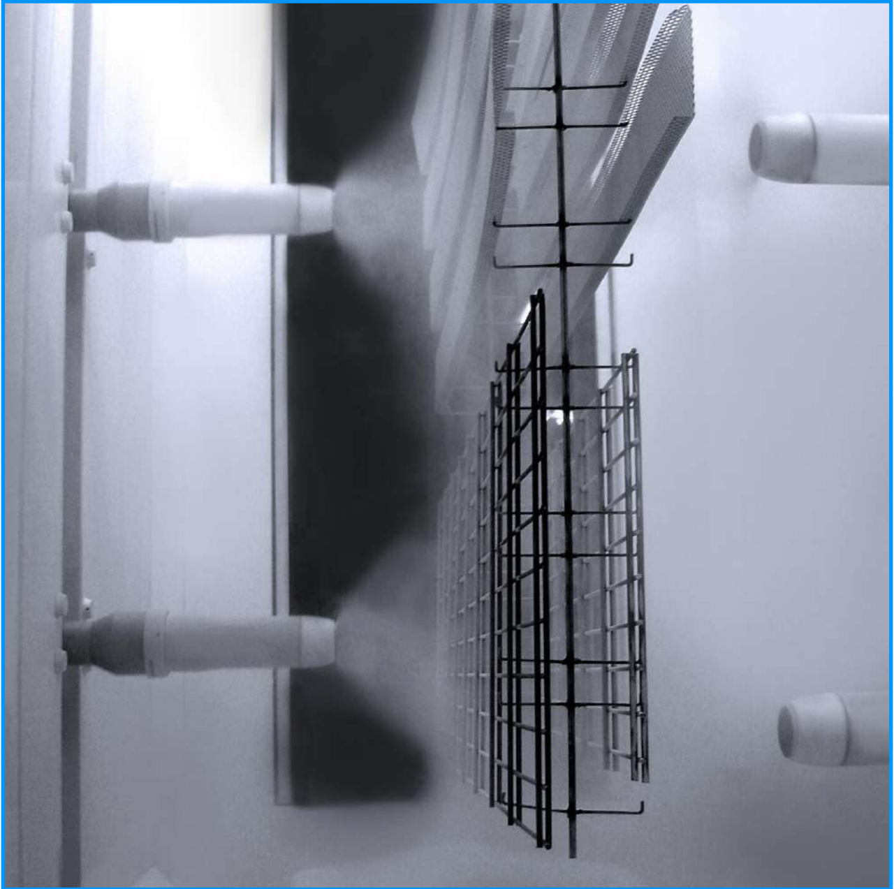
ตัวอย่างการติดตั้งกับแขนกลแนวตรง Example of attaching with reciprocator
