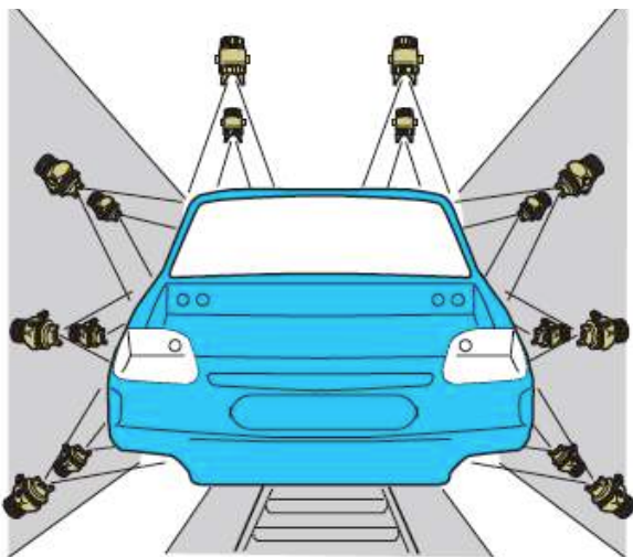
ใช้พ่นน้ำยากันสะเก็ดสำหรับตัวถังรถยนต์ได้ Applying Spatter-Prevention Liquid
