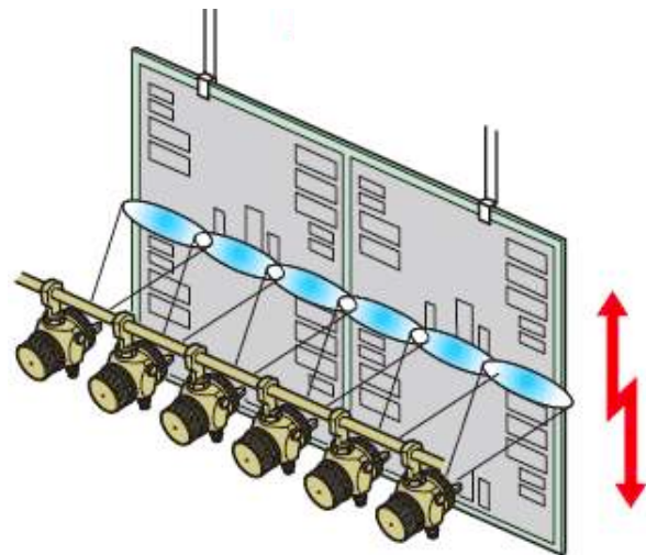
ใช้พ่นตัวต้านในฉนวนไฟฟ้าบนแผงวงจรในระหว่างการผลิต Applying resist material to electrically insulate printed circuit boards during manufacturing
