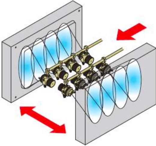
ใช้พ่นน้ำยาลอกแบบบนเครื่องฉีดโลหะเหลวสำหรับหล่อแบบ Applying mold release on die-casting machines
