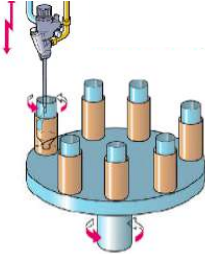
ใช้พ่นภายในชิ้นงานทรงกระบอก Applying to inside of cylinders
