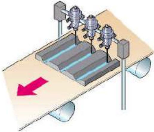
พ่นกาวลงบนร่องตัววี Applying adhesive to v grooves
