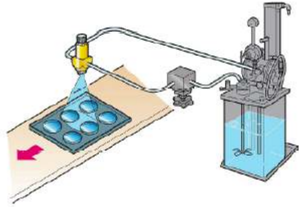
ใช้พ่นน้ำยากันรอยขีดข่วนบนเลนส์ Applying scratch prevention agent on lenses
