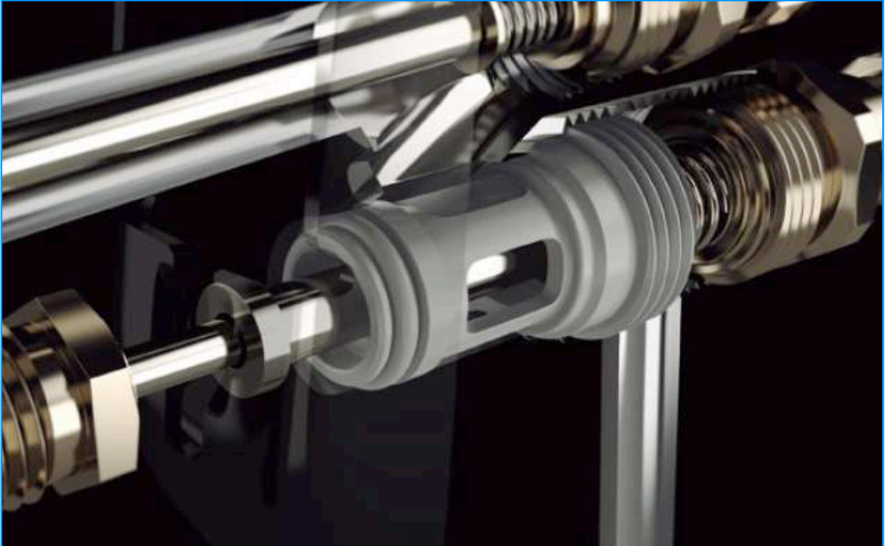
ตำแหน่งช่องทางลำเลียงลม Position of Air channel
